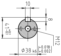
SEZ. A-A
