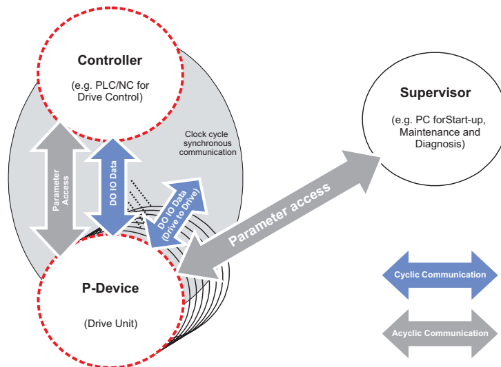
Fig. 5.1.6: Presentazione dei servizi di comunicazione disponibili tra i dispositivi PROFdrive
