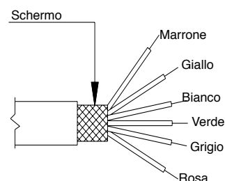
F - Cavo 6 poli
