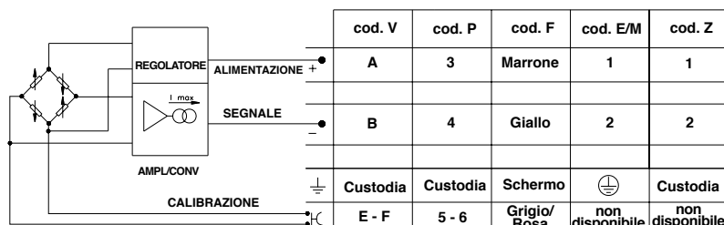
USCITA AMPLIFICATA IN CORRENTE - mod. E
