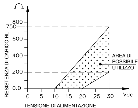
DIAGRAMMA DI CARICO (Uscita corrente)
