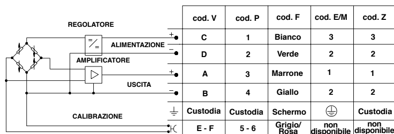
USCITA AMPLIFICATA IN TENSIONE - mod. B/C/M/N/P/Q/R
