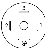
E - Conn. 4 poli EN 175301-803A M - Conn. 4 poli EN 175301-803C
