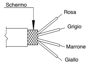
F - Cavo 4 poli
