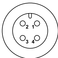
Z - Connettore maschio 4 poli M12 x 1
